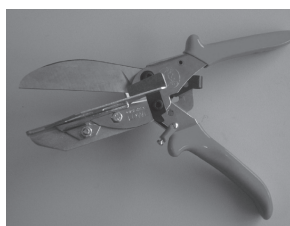
Cisaille à onglet démultipliée Référence : Janser : 262 284 000 Pour découpe autour des pieds d'huisserie, endroits difficiles d'accès.
